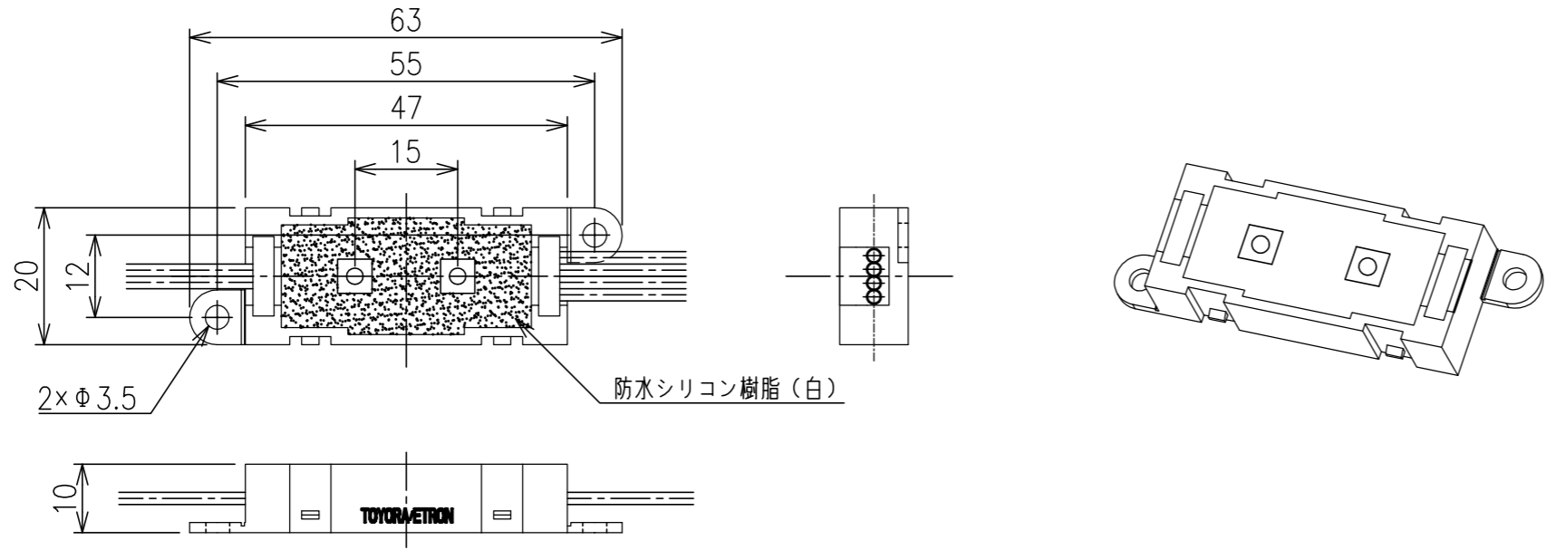
モジュール本体詳細図 (S=1/1)
